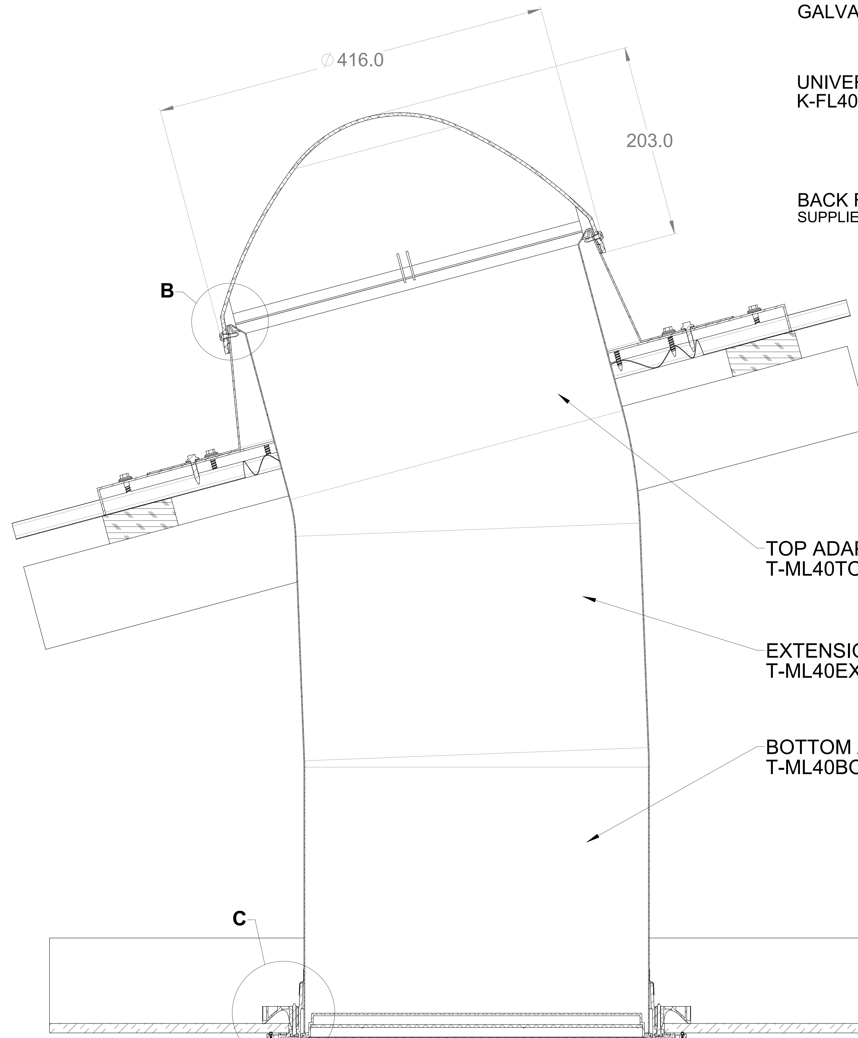
SECTION SCALE 1 : 2
